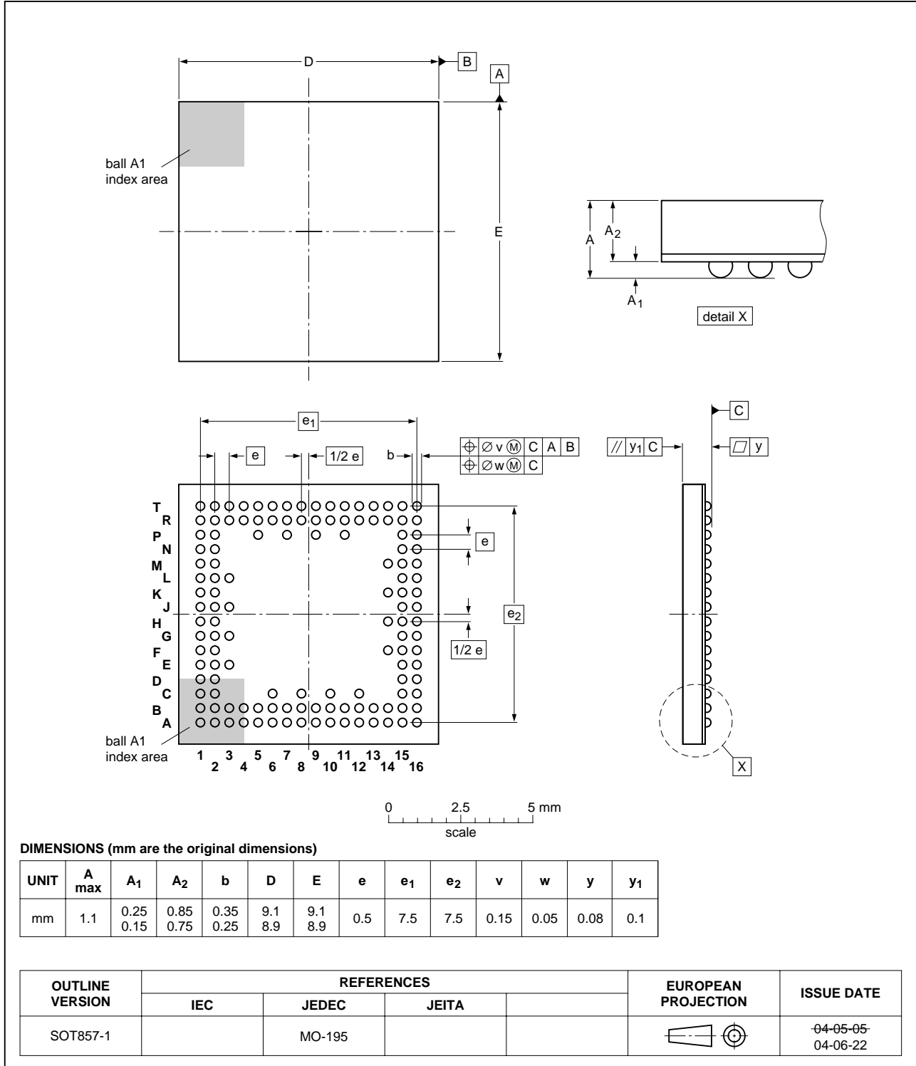
SOT857-1
